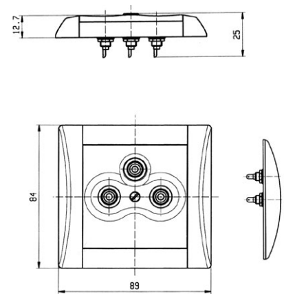
zásuvka AUDIO-VIDEO
