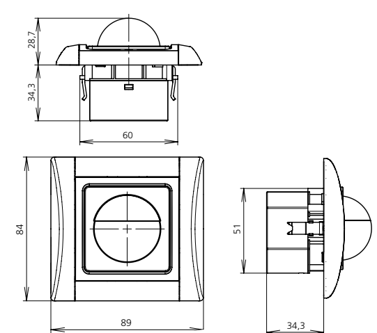
pohybové čidlo B.E.G.
