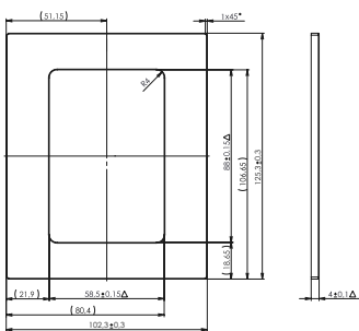
rámeček dvojzásuvky
