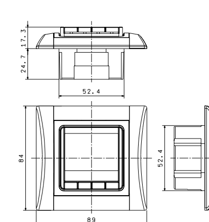
digitální termostat DSE 4T
