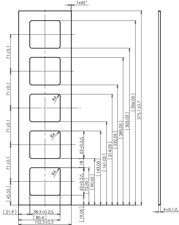
rámeček pětínásobný svislý
