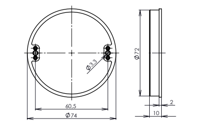
vymezovací kroužek VK1
