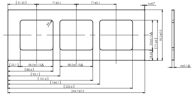
rámeček čtyřnásobný vodorovný
