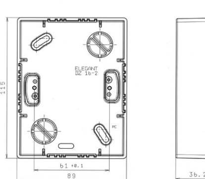
elektroinstalační krabice pro lištové rozvody pro dvojzásuvku
