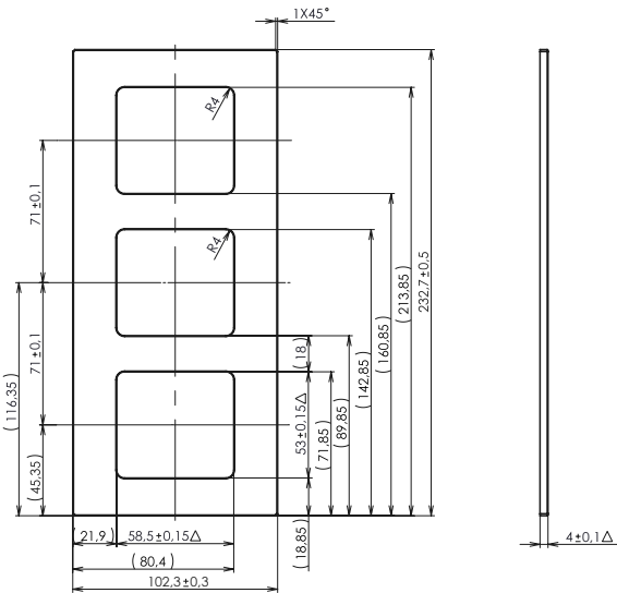
rámeček trojnásobný svislý
