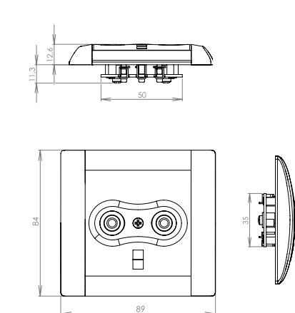
zásuvka ochranného pospojování
