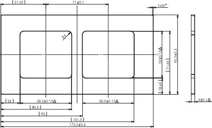
rámeček dvojnásobný vodorovný
