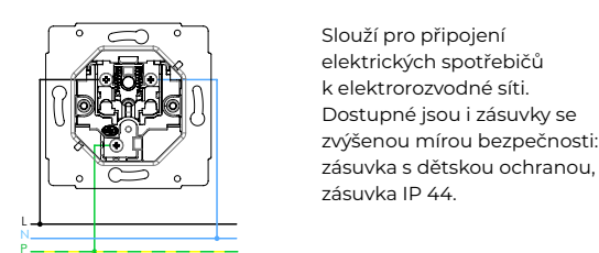
zásuvka jednonásobná
