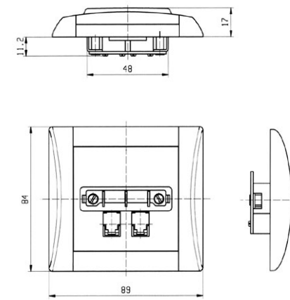
zásuvka telefonní
