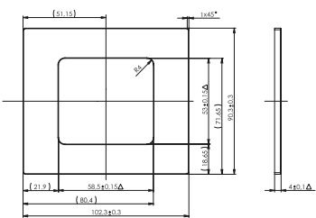
rámeček jednonásobný
