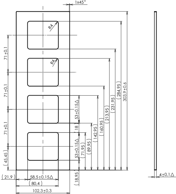
rámeček čtyřnásobný svislý
