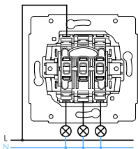
spínač řazení 1+1+1
