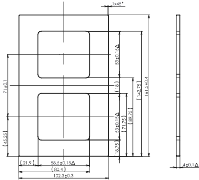
rámeček dvojnásobný svislý
