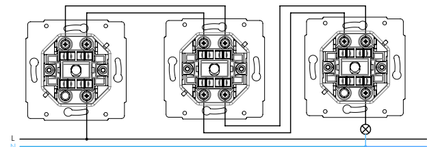
spínač řazení 6+7+6 střídavý - křížový - střídavý přepínač
