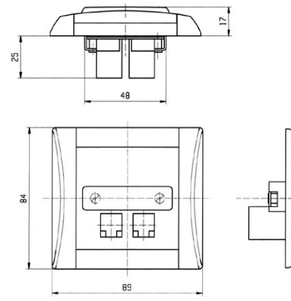
zásuvka komunikační
