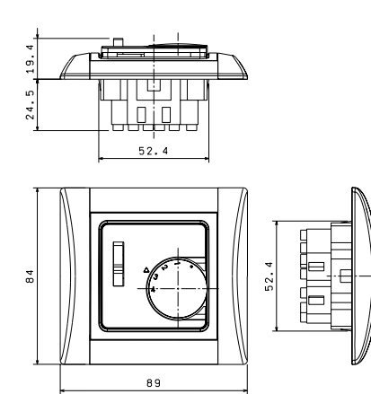
analogový termostat OREG/EBERLE DSE 2T/3T
