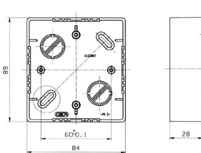
elektroinstalační krabice pro lištové rozvody
