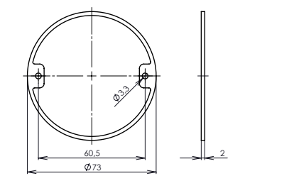
vymezovací kroužek VK2
