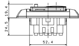
analog thermostat OREG/EBERLE DSE 2T/3T
