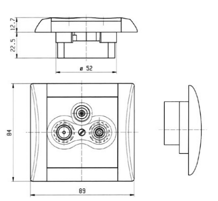
TV+R+SAT sockets
