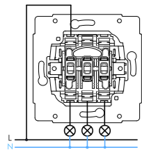
switch arrangement 1+1+1
