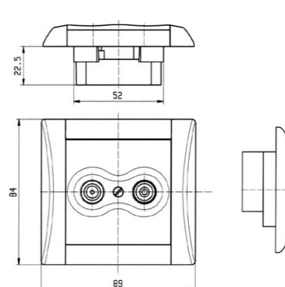
TV+R sockets
