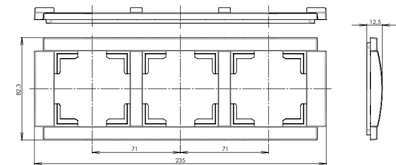
rámeček trojnásobný, vodorovný
