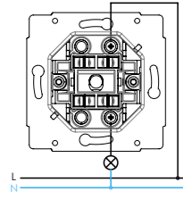
spínač řazení 1+1+1
