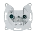
zásuvka TV+R průběžná odbočovací útlum 9 dB pro koaxiální kabely průměru 4,5–8,3 mm typové označení na výrobku: ZAP 9/K
