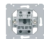
přístroj řízení 7 přepínač křížový 10 AX, 250 V AC
