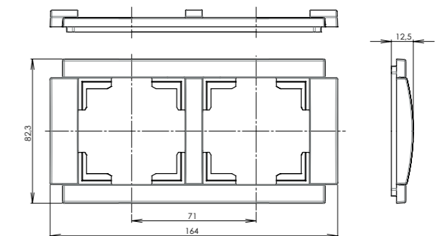
rámeček dvojnásobný
