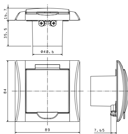
zásuvka vysavačová
