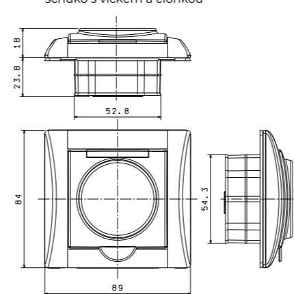
zásuvka IP 44 jednonásobná/ schuko s víčkem a clonkou
