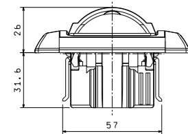
pohybové čidlo STEINEL
