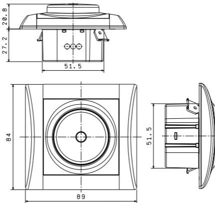
strmívač otočný s tlačítkovým spínačem PUSH-PULL a funkcí řazení č. 6
