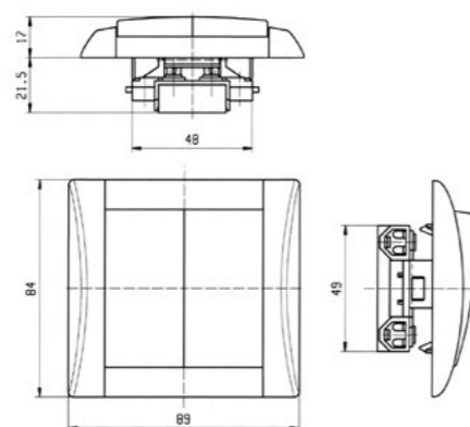
spínač s dvojitým krytem
