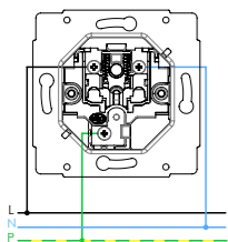
zásuvka jednonásobná
