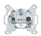
zásuvka TV+R+SAT průběžná, útlum 10 dB, 300 mA, 24 V DC pro koaxiální kabely průměru 4,5–8,3 mm typové označení na výrobku: ZAR-SAT 10/P3
