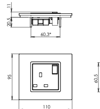
zásuvka jednonásobná
