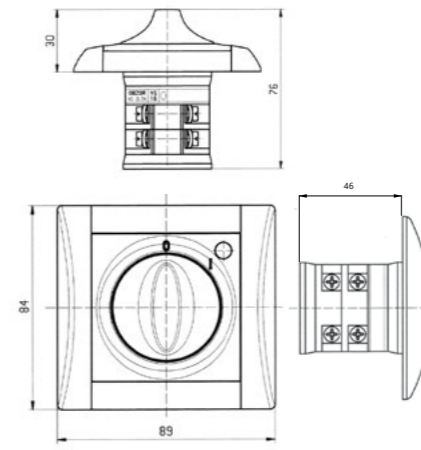
sporákový spínač otočný
