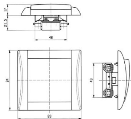
spínač s jednoduchým krytem
