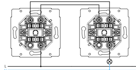
spínač řazení 6 schodišťový vypínač (střídavý přepínač), jednopolový dvoucestný přepínač bez polohy vypnuto
