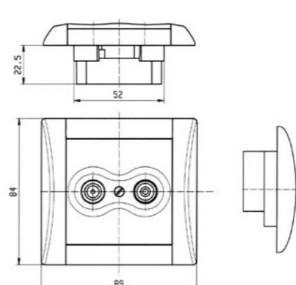
zásuvka TV+R
