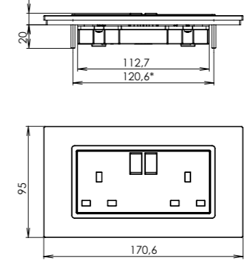
zásuvka dvojnásobná
