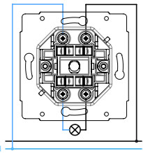
spínač řazení 2 (dvoupólový vypínač)
