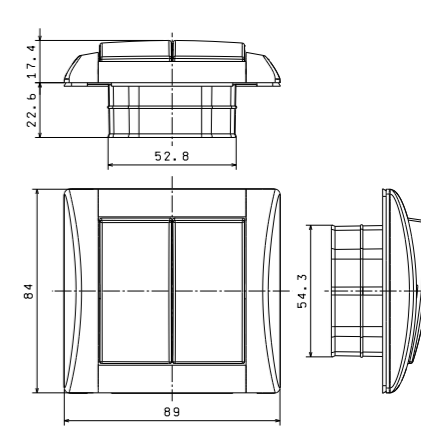
spínač IP 44 s dvojitým krytem
