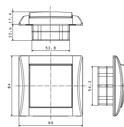
spínač IP 44 s jednoduchým krytem
