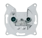
zásuvka TV+R průběžná odbočovací útlum 14 dB pro koaxiální kabely průměru 4,5–8,3 mm typové označení na výrobku: ZAP 14
