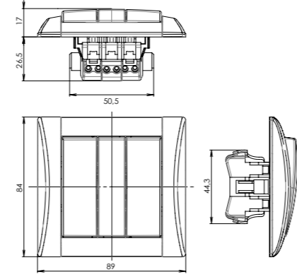
spínač s trojitým krytem
