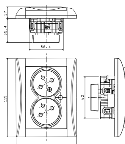
zásuvka dvojnásobná s přep. ochranou a clonkou
