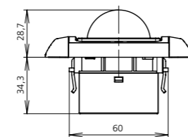
pohybové čidlo B.E.G.
