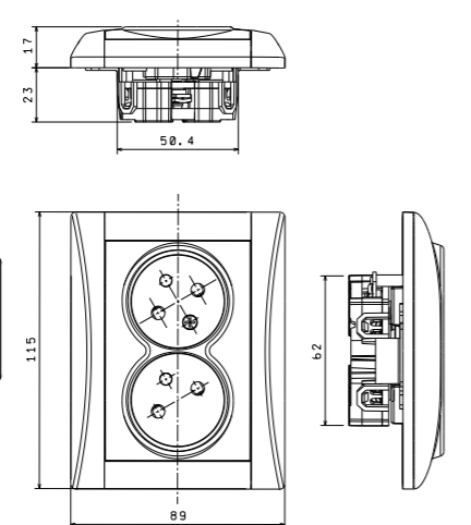
zásuvka dvojnásobná s (bez) clonkou
