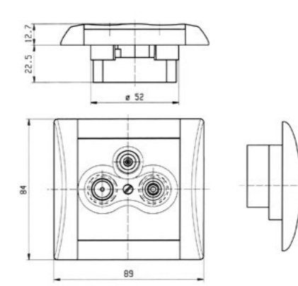
zásuvka TV+R+SAT
