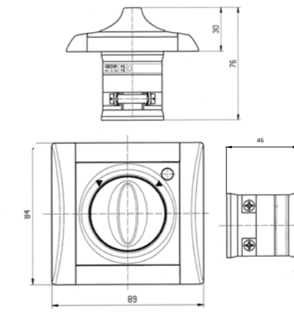
žaluziový ovladač
